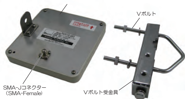
アンテナ (PAT511S-4953)
