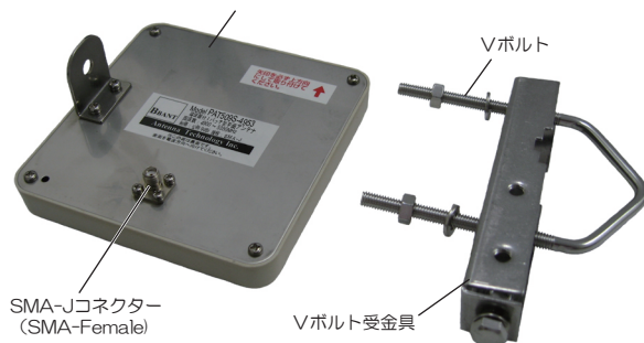
アンテナ (PAT509S-4953)
