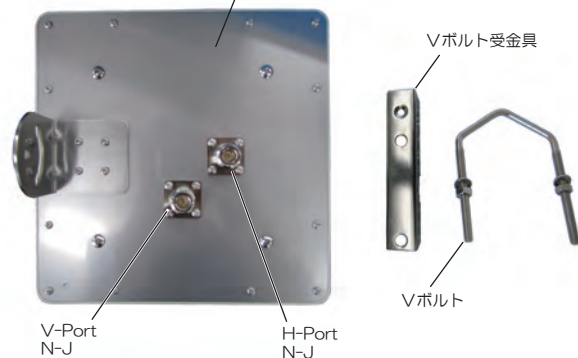
アンテナ (PAT214H-NX2-24)
